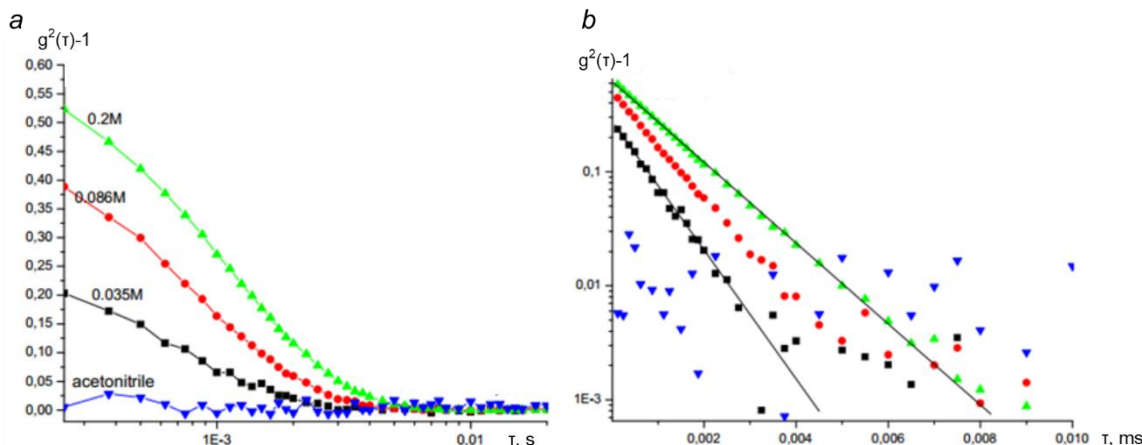
Рис. 1. Данные динамического рассеяния света (ДРС), корреляционные функции для растворов метил(фенил-5-трифторацетоамид-4,7,8,9-тетра- O -ацетил-3,5-дидезокси-2-тио- D -глицеро- \beta - D -галактононулопиранозид)оната в безводном ацетонитриле с концентрациями: черные квадраты – 0.035 моль/л, красные круги – 0.086 моль/л, зеленые треугольники – 0.2 моль/л, синие обратные треугольники – чистый ацетонитрил.
